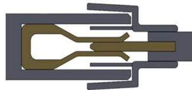
&lt;단면도&gt;
